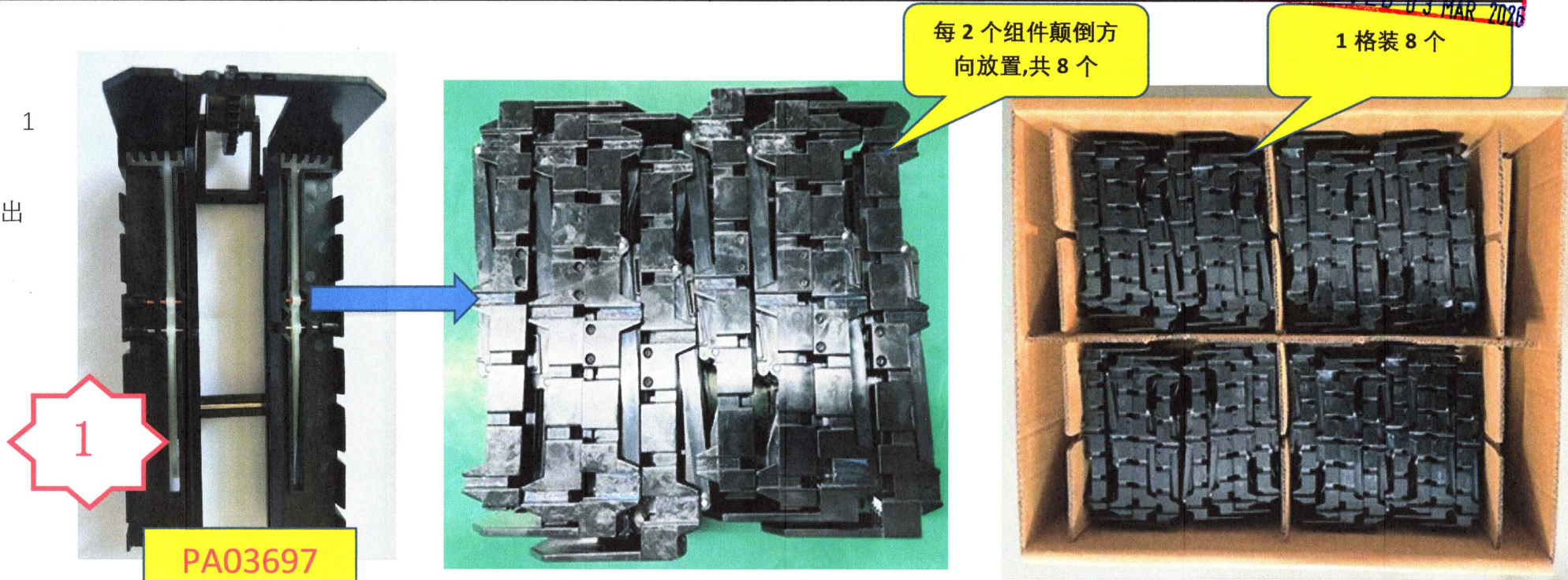
图一，将 PA03697 每 2 个组件颠倒方向放置，按图示放入，1 格装 8 个组件，1 层 4 格共 32 个，1 箱有两层共 64 个，注意底层，中层，最上层需各放置 1 块大隔板。
